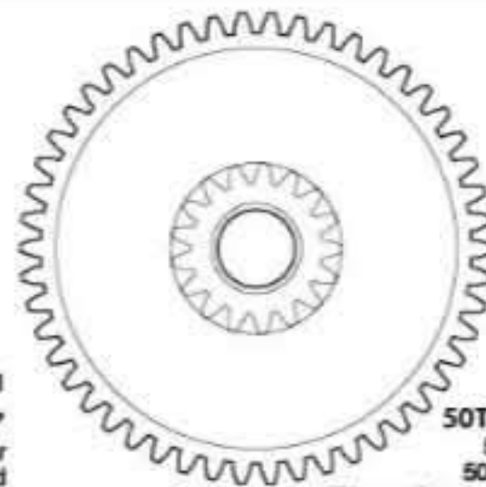
GB3 x1 デフキャリア Differential spur gear Differentialrad Couronne de différentiel
