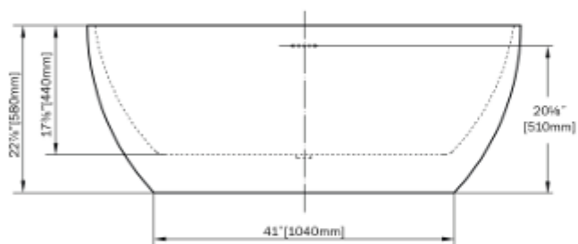
FRONT VIEW - VUE DE FACE
