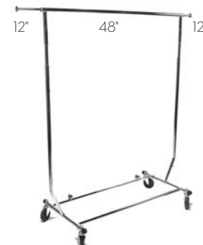
2901 Penderie droite ajustable, sur roues, structure en tube carré de 1", pôle ronde Adjustable single hangrail rolling rack 1" square tubing, round hangrail 60" x 20" x 54" à 74" H
